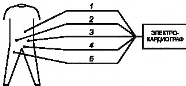
Рисунок ВВ.1а — Отведения и их цвет кодировки при регистрации ЭКГ плода (см. таблицу ВВ.1, 6.1)
