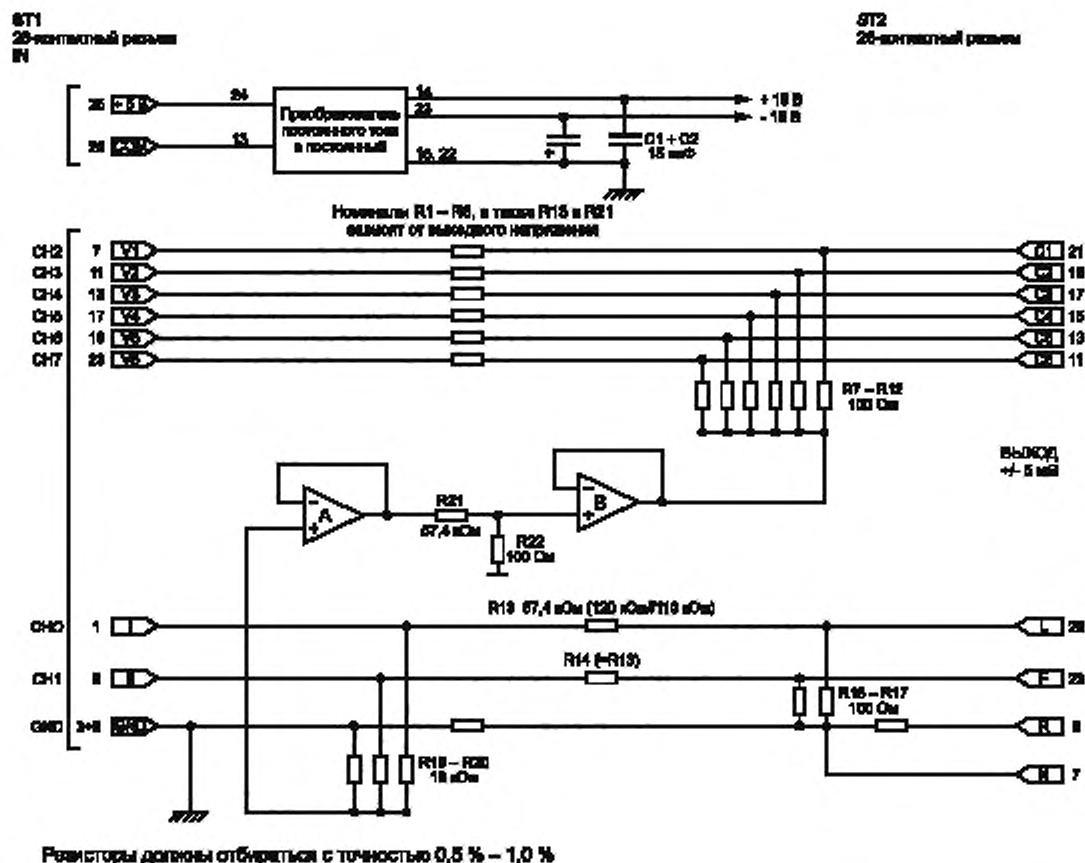
Рисунок II.2 — Пример схемы предварительной обработки ЭКГ-сигналов
