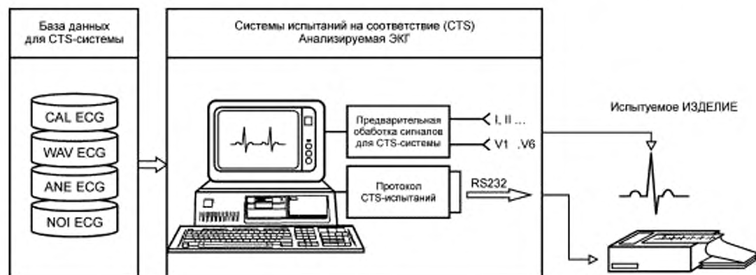
Рисунок II.1 — Система испытаний изделия на соответствие (CTS-система)
