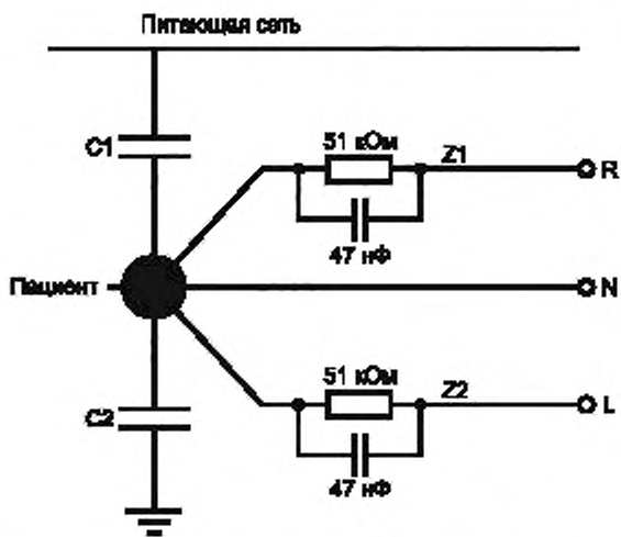
Рисунок FF.1 — Эквивалентная электрическая схема ПАЦИЕНТА, подключенного к ЭЛЕКТРОКАРДИОГРАФУ
