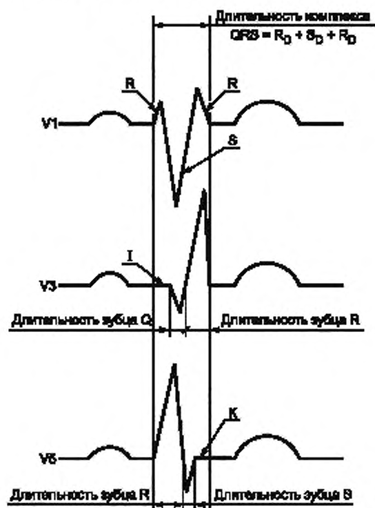
Рисунок GG.3 — Длительности зубцов, изоэлектрические сегменты
