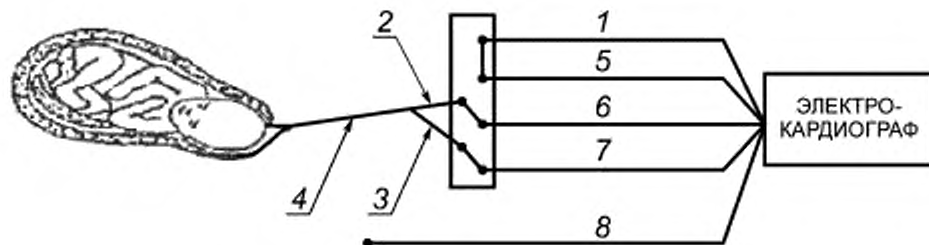
Рисунок ВВ.2 — Положение и цвет кодировки ЭЛЕКТРОДОВ на головке плода (см. таблицу ВВ.1, 6.1)
