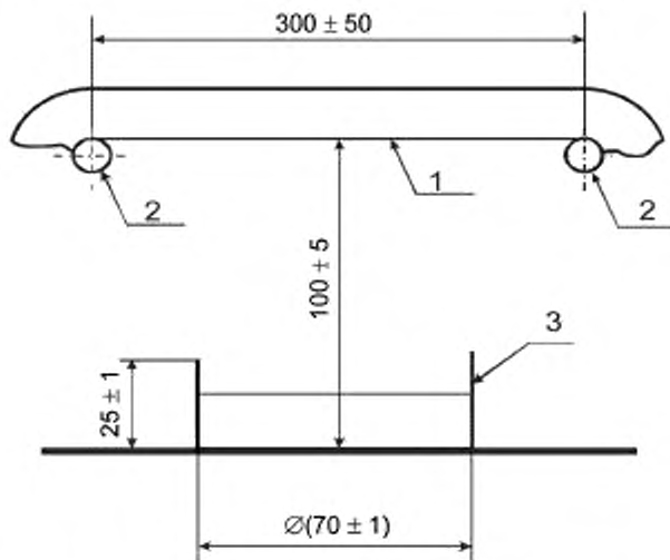
1 — испытываемый образец (тетивы, ступеньки); 2 — опоры; 3 — емкость для горючего
