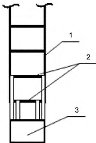
Рисунок 4 — Испытание лестницы на прочность
