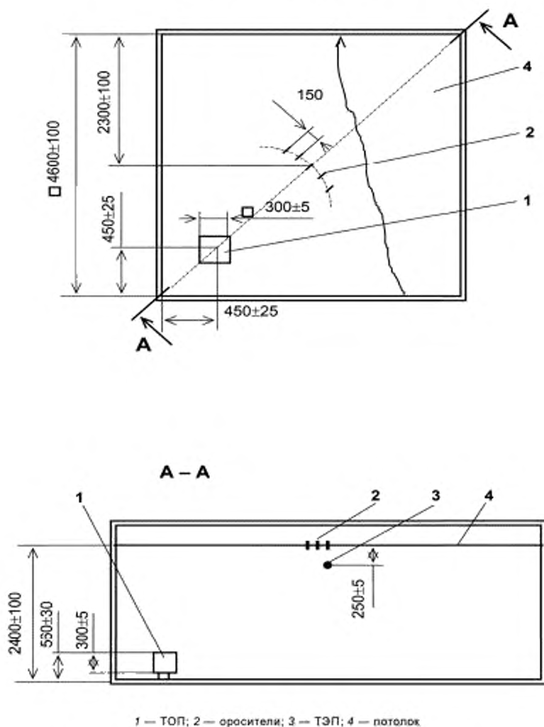
Рисунок Б.1 — Расположение оросителей, ТОП и ТЭП в испытательном помещении
