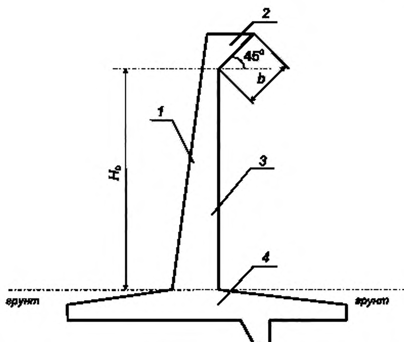
Рисунок А.1 — Принципиальная схема ограждающей стены с волноотражающим козырьком
