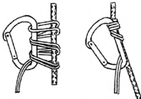
Рисунок 10 — Узел Бахмана
