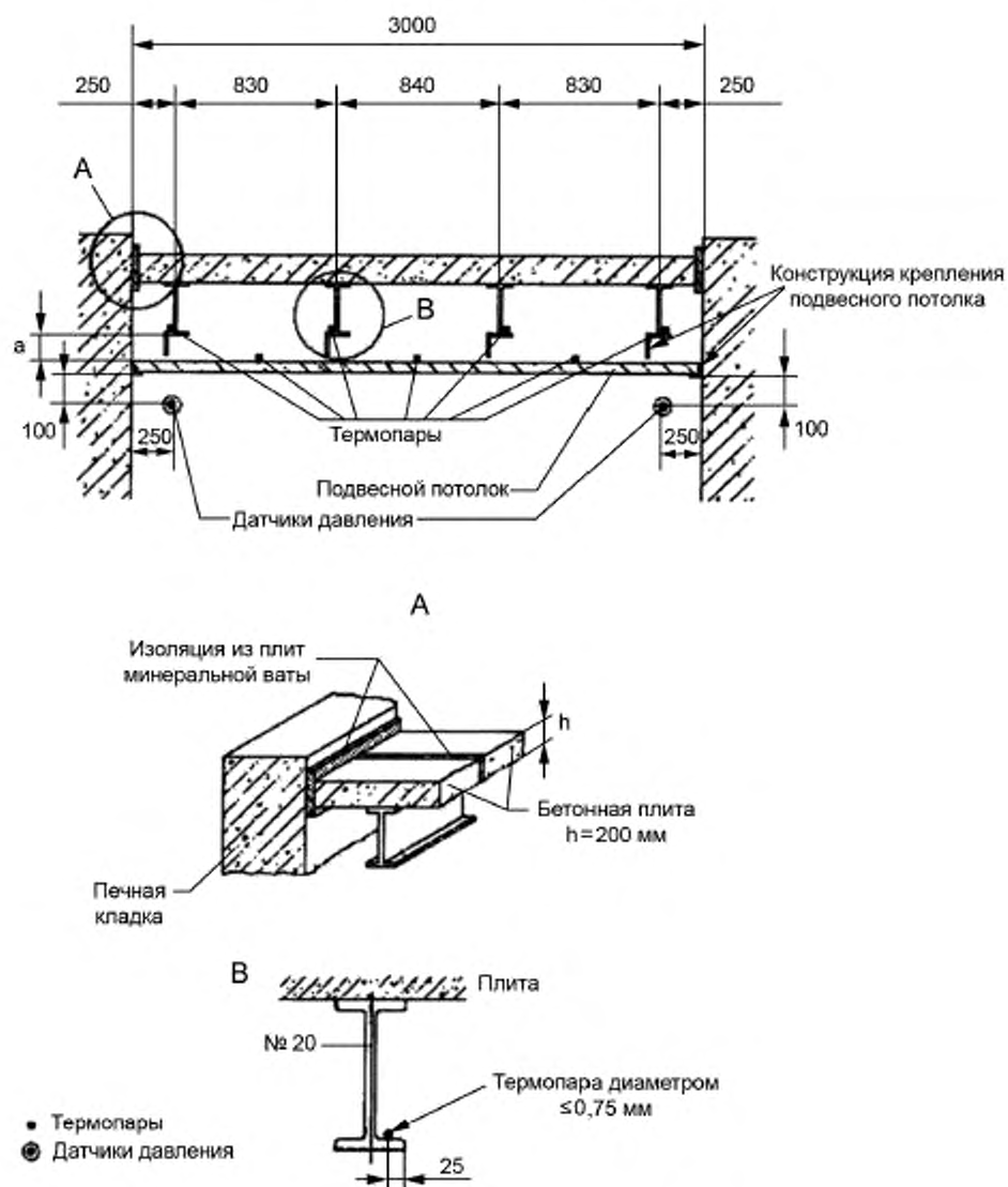
Рисунок А.1 — Схема испытательного блока
