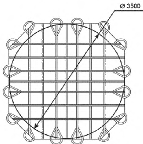
Рисунок 1 — Конструкция ПСН
