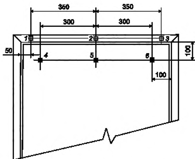
1, 3, 4, 6 — термодатчики устанавливаются обязательно; 2, 5 — термодатчики не устанавливаются, если размеры между термодатчиками меньше указанных на рисунке
