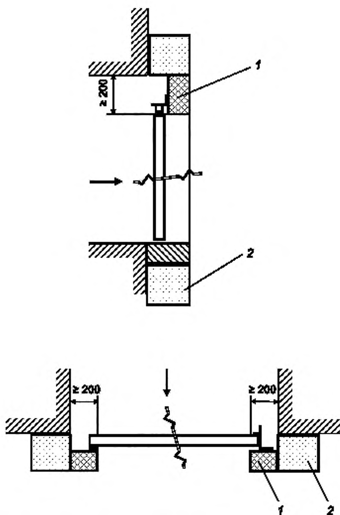
1 — фрагмент ограждающей конструкции; 2 — рама для установки фрагмента ограждающей конструкции; →, ↓ — направление теплового воздействия
