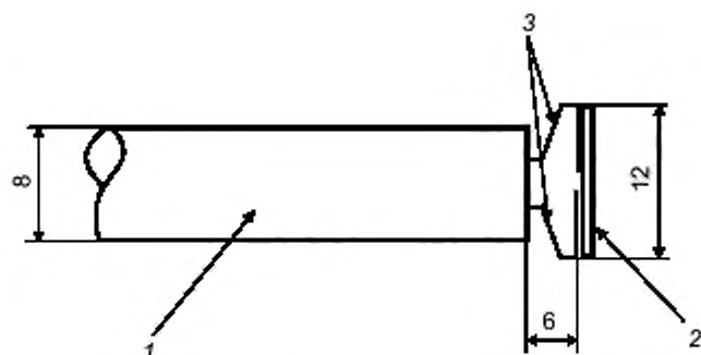
1 — двухканальная керамическая трубка; 2 — медный диск толщиной 0,5 мм; 3 — термопарные провода диаметром 0,7 мм
