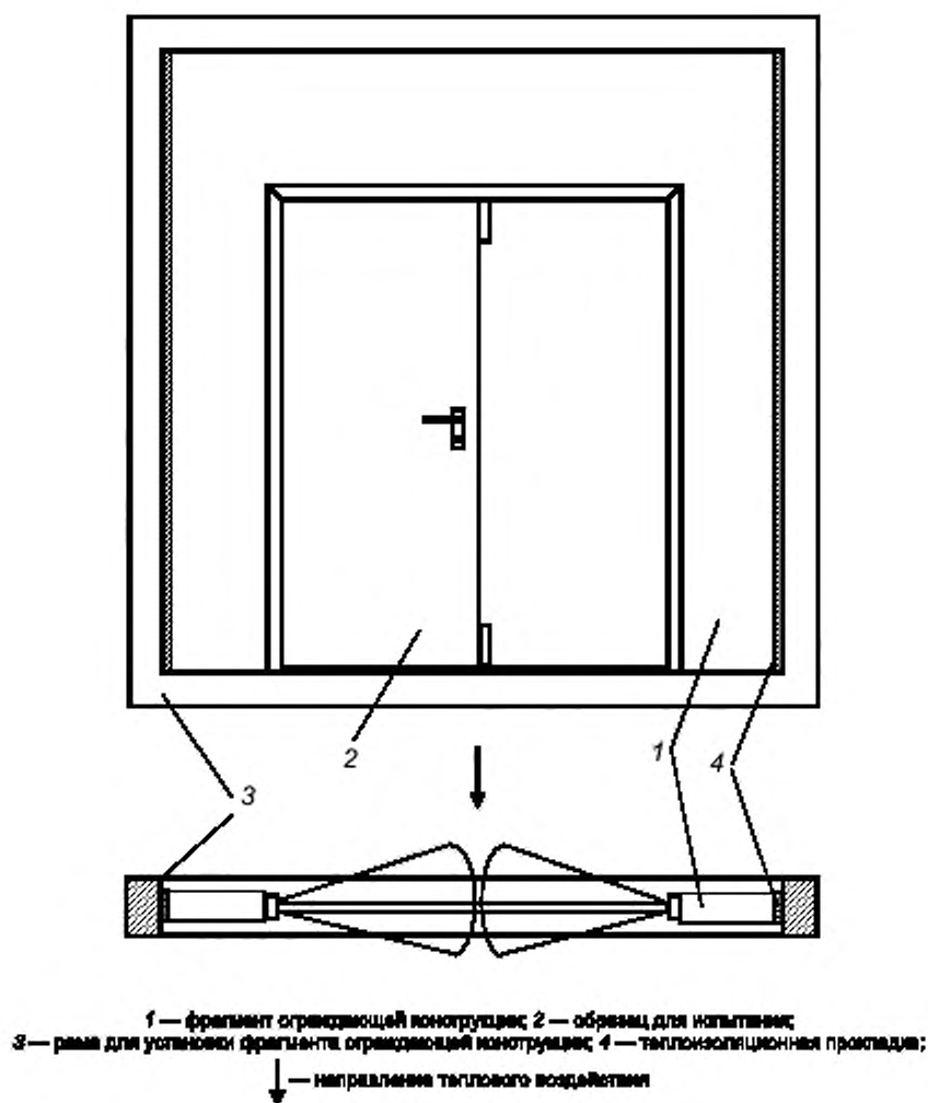
Рисунок 4 — Конструкция двери в гибком фрагменте ограждающей конструкции
