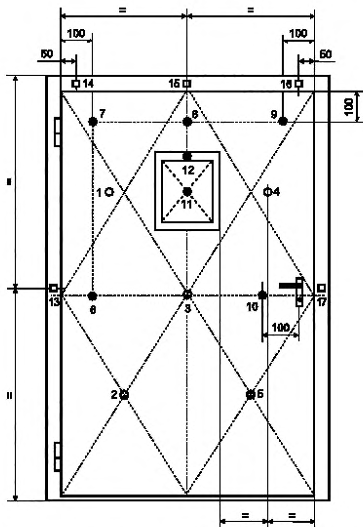
Рисунок 21 — Схема установки термодатчиков на необогреваемой поверхности распашной одностворчатой двери с частичным остеклением
