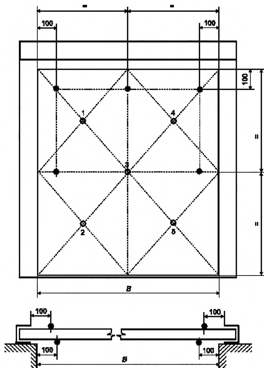
Рисунок 16 — Схема установки термоплат на необогреваемых поверхностях полотен подъемных и скручивающихся ворот
