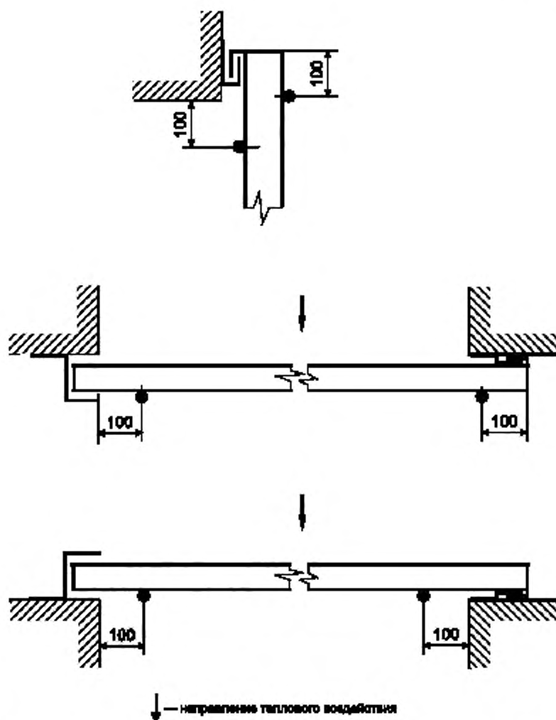
Рисунок 15 — Схема установки термистора на неогреваемой поверхности полотна откатной двери (ворот) в зоне 100 мм от его торцевых поверхностей, края, коробки и проема в свету
