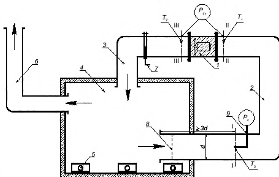
1 — испытуемый образец вентилятора; 2 — всасывающий воздуховод; 3 — нагнетательный воздуховод; 4 — печь; 5 — форсунки; 6 — дымоход; 7 — дросселирующее устройство; 8 — выравнивающее устройство; 9 — комбинированный приемник давления (КПД); I—I, II—II, III—III — мерные сечения; ТЭП — термоэлектрический преобразователь (ТЭП); T_1 , T_2 , T_3 — температуры на входе и выходе из вентилятора и в сечении измерения расхода газов соответственно; P_{ст} — статическое давление вентилятора; P_c — перепад давления на КПД
