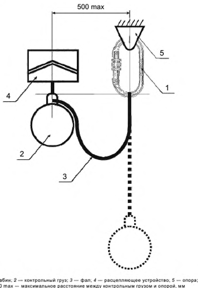
Рисунок 5 — Схема испытания карабина на динамическую прочность
