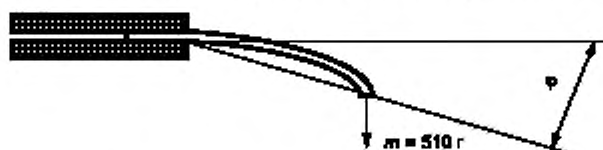
Рисунок 4 — Схема измерения угла сгиба
