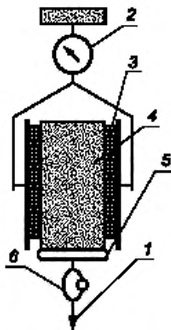
1 — место приложения нагрузки; 2 — датчик силы (динамометр); 3 — ролик; 4 — пояс; 5 — карабидержатель; 6 — карабин пожарный
