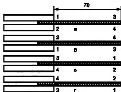
Рисунок 3 — Положения зажима образца ленты
