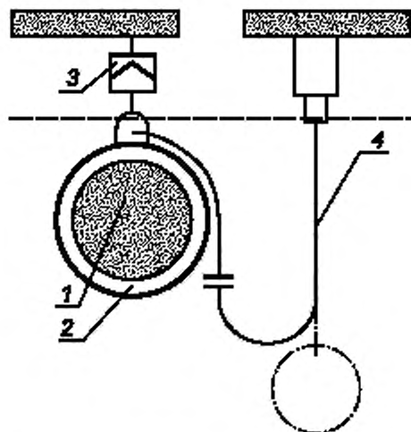
1 — груз; 2 — пояс; 3 — расцепляющее устройство; 4 — канат стальной
