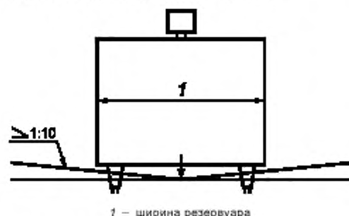
Рисунок 2 — Зазор между резервуаром и полом
