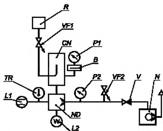
CN — измерительная камера; ND — испытуемый насос; P1, P2 — вакуумметры; B — охлаждаемая ловушка; VF1, VF2 — клапаны-напечатели; V — клапан; R — устройство для измерения потока; L1 — измеритель расхода воды; L2 — измеритель мощности; N — насос форвакуумный; TR — датчик измерения температуры
