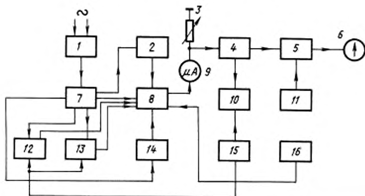
Структурная схема испытательной установки
