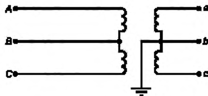
А, В, С — фазы первичной обмотки ТН; а, b, с — фазы основной вторичной обмотки ТН
