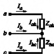
а, b, с — фазы основной вторичной обмотки ТН; I_a, I_b, I_c — фазные токи; I_{ab}, I_{bc} — междофазные токи; Z_{ab}, Z_{bc} — междофазные нагрузки
