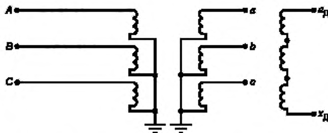
А, В, С — фазы первичной обмотки ТН; а, b, с — фазы основной вторичной обмотки ТН; x_d , x_d — фазы дополнительной вторичной обмотки ТН
