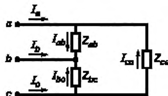
а, b, с — фазы основной вторичной обмотки ТН; I_a, I_b, I_c — фазные токи; I_{ab}, I_{bc}, I_{ca} — междофазные токи; Z_{ab}, Z_{bc}, Z_{ca} — междофазные нагрузки
