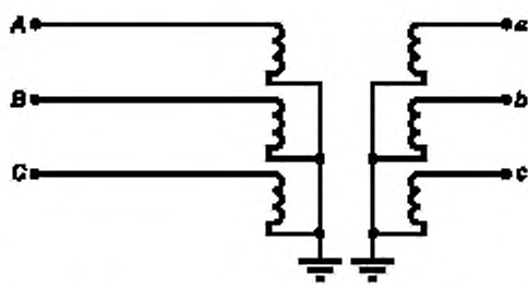
А, В, С — фазы первичной обмотки ТН; а, b, с — фазы основной вторичной обмотки ТН
