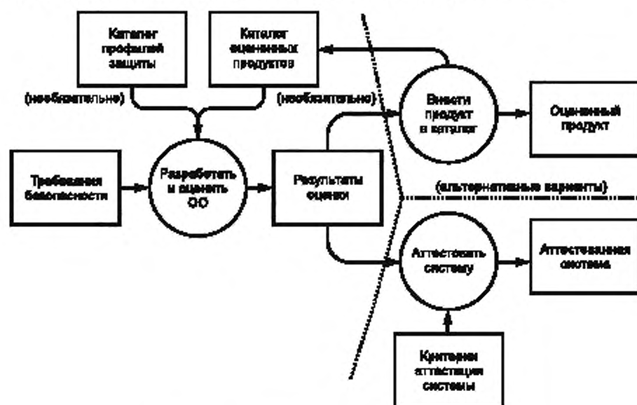
Рисунок 10 — Использование результатов оценки ОО
