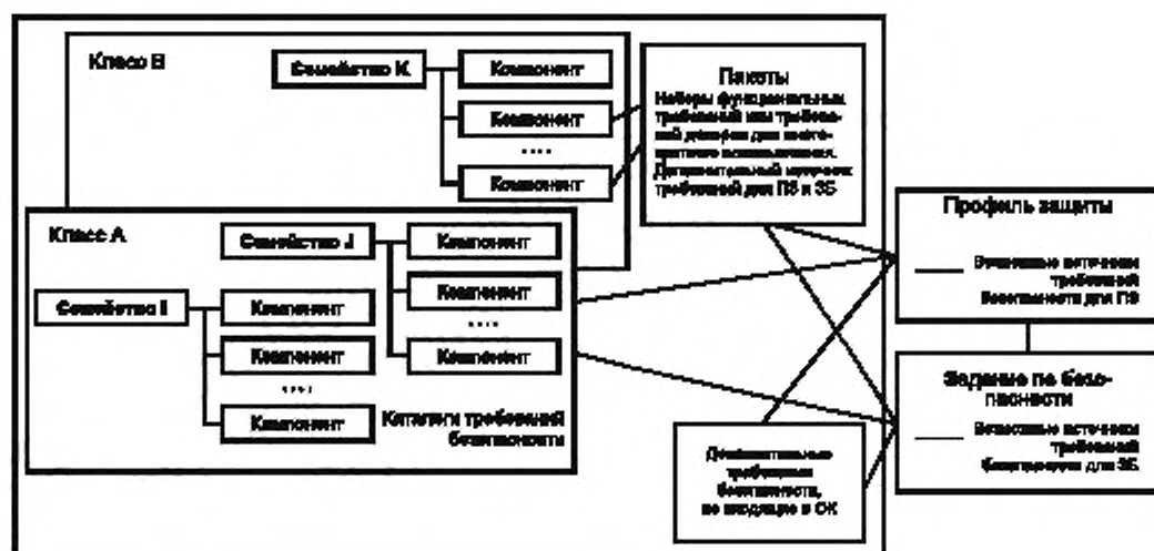
Рисунок 7 — Организация и структура требований
