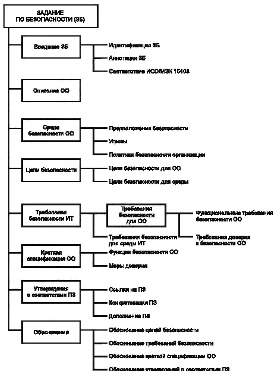
Рисунок В.1 — Содержание задания по безопасности
