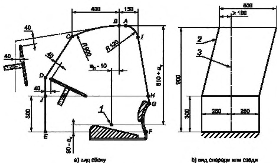
Рисунок 6 — Объем ограничения деформации
