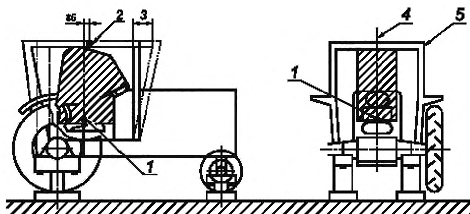
1 — СИР; 2 — точка приложения силы сбоку (см. 7.2.3); 3 — деформация под воздействием приложения силы сзади; 4 — продольная плоскость симметрии; 5 — сила сбоку
