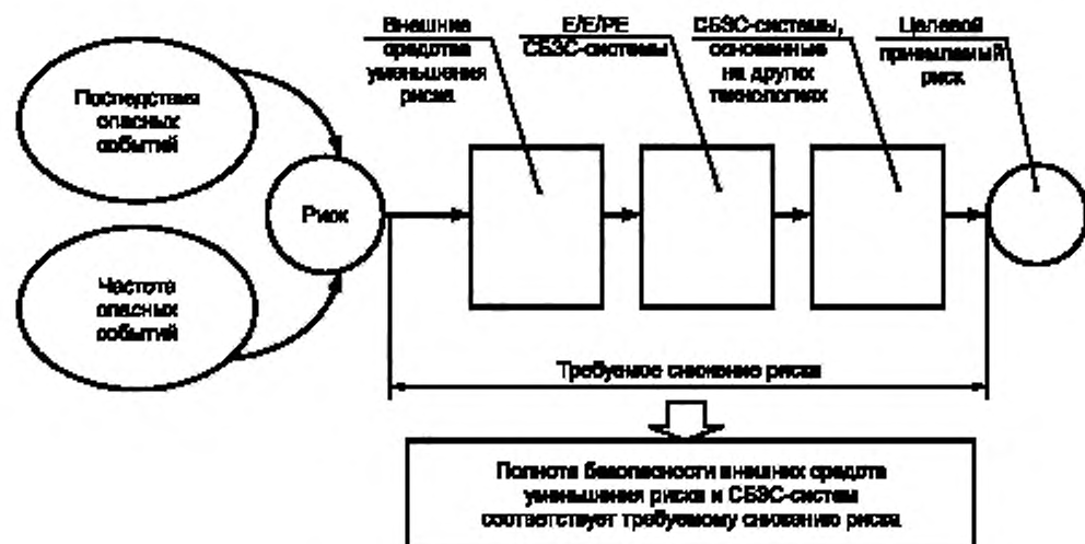
Рисунок Е.2 — Риск и полнота безопасности
