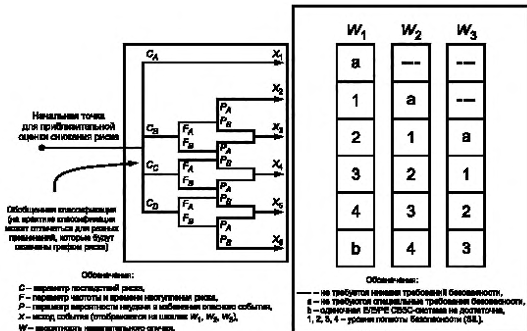
Рисунок Ж.1 — Общая схема графа риска
