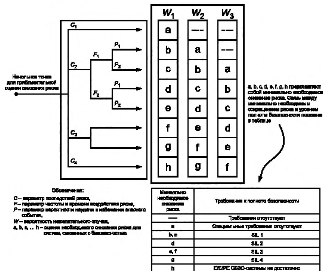
Рисунок Ж.2 — Пример реализации графа риска
