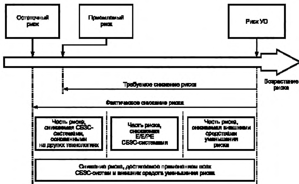
Рисунок Е.1 — Общий подход к снижению риска
