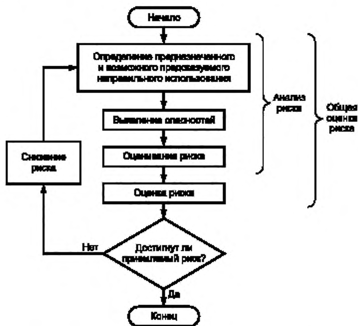
Рисунок 2 — Итеративный процесс общей оценки и снижения риска
