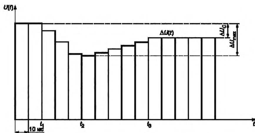
Рисунок 2 — Схема определения огибающей среднеквадратических значений напряжения
