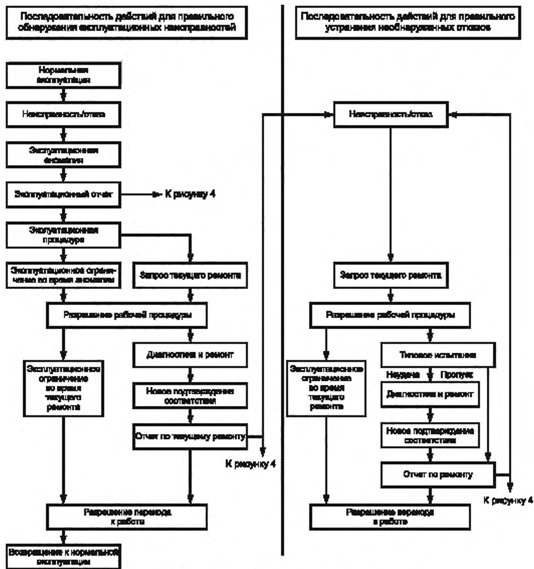
Рисунок 3 — Пример модели эксплуатации и текущего ремонта
