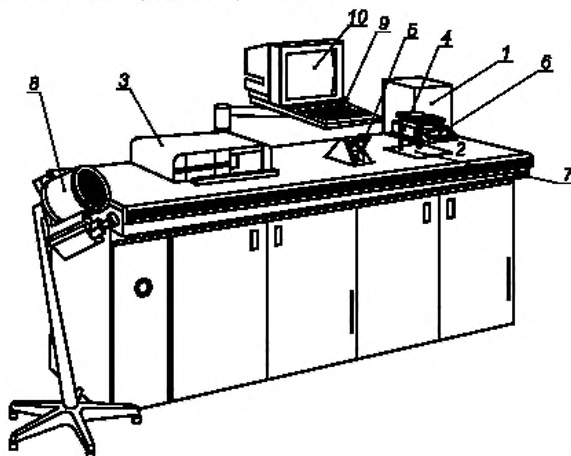
1 — модуль микронейра; 2 — модуль цвета/сора; 3 — модуль длины/прочности; 4 — плата для прижима пробы к поверхности окна во время измерений показателей цвета и засоренности хлопкового волокна; 5 — камера микронейра; 6 — электронные весы; 7 — световое окно для размещения пробы при измерении показателей цвета и засоренности хлопкового волокна; 8 — фибросэмплер; 9 — алфавитно-цифровая клавиатура; 10 — монитор
