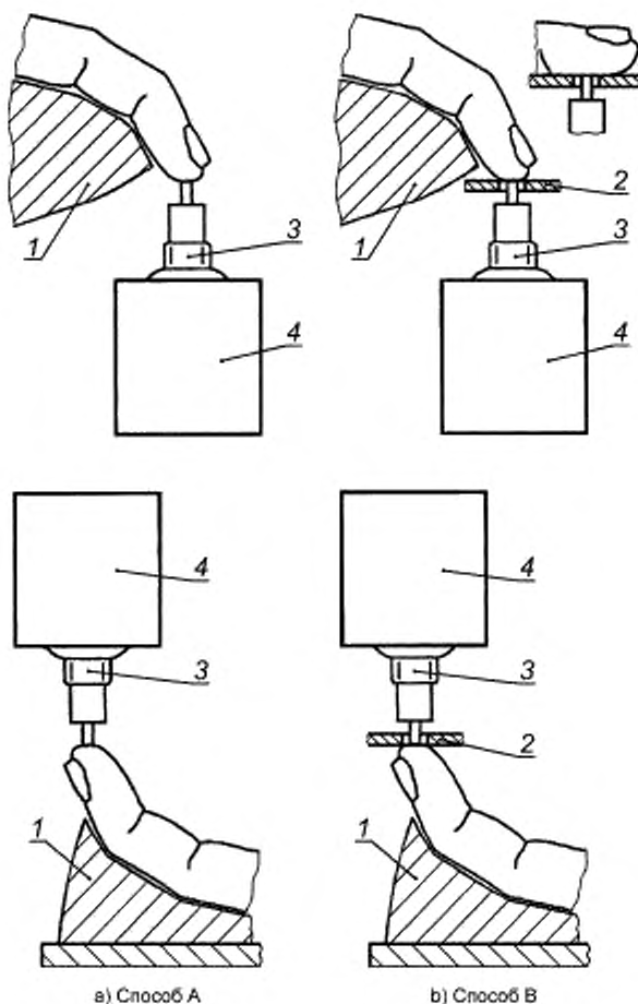
1 — опора пальца; 2 — подставка; 3 — датчик; 4 — стимулятор
