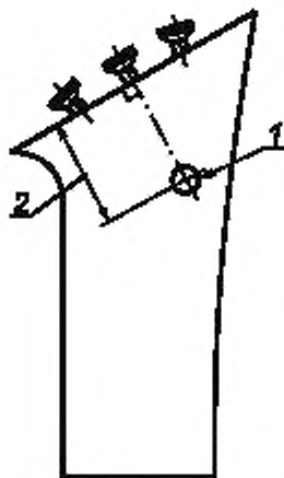
1 — просверленное технологическое отверстие под стержень диаметром 2 мм. 2 — расстояние от верхней части каблука до технологического отверстия от 20 до 25 мм
