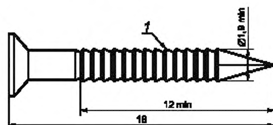
Рисунок 1 — Стандартный каблучный гвоздь
