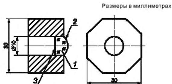
1 — эталонная линза; 2 — тороидальная поверхность; 3 — плоская поверхность
