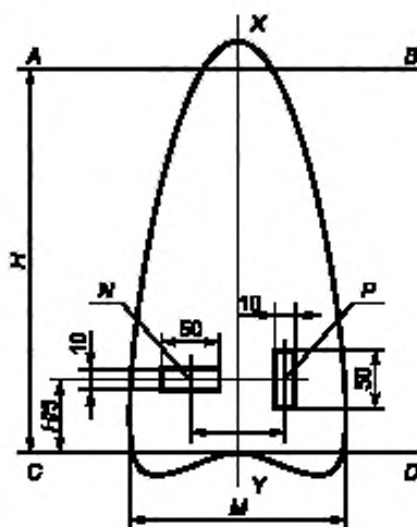
Рисунок 10 — Разметка шкур нутрии и норки
