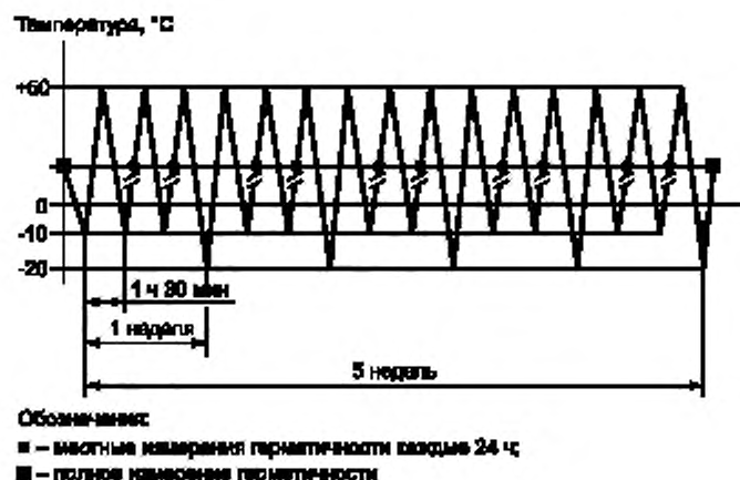
Рисунок И.2 — Термоциклирование
