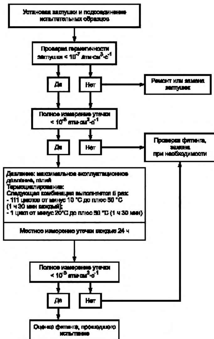
Рисунок И.1 — Испытание фитинга на герметичность
