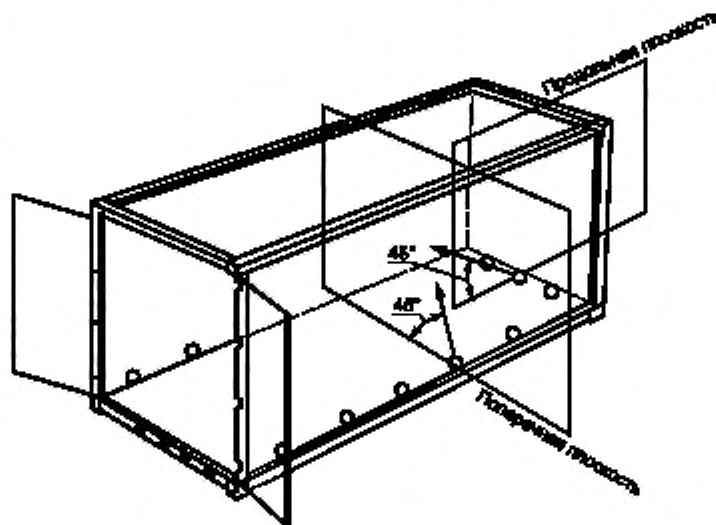
Рисунок Е.1 — Схема приложения испытательных нагрузок
