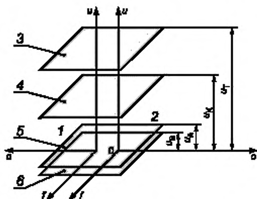
1 — правая; 2 — левая; 3 — верхняя базовая плоскость T; 4 — коленная базовая плоскость K; 5 — голеностопная базовая плоскость A; 6 — нижняя базовая плоскость B
