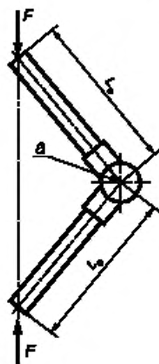
L_0 — длина узлов бедра и голени; a — действительный центр коленного узла
