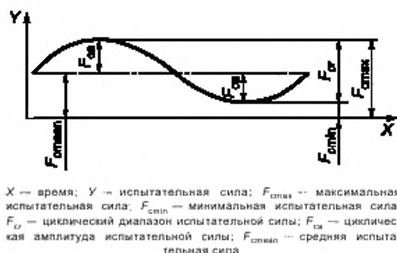
Рисунок 9 — Параметры нагружения при основном циклическом испытании
