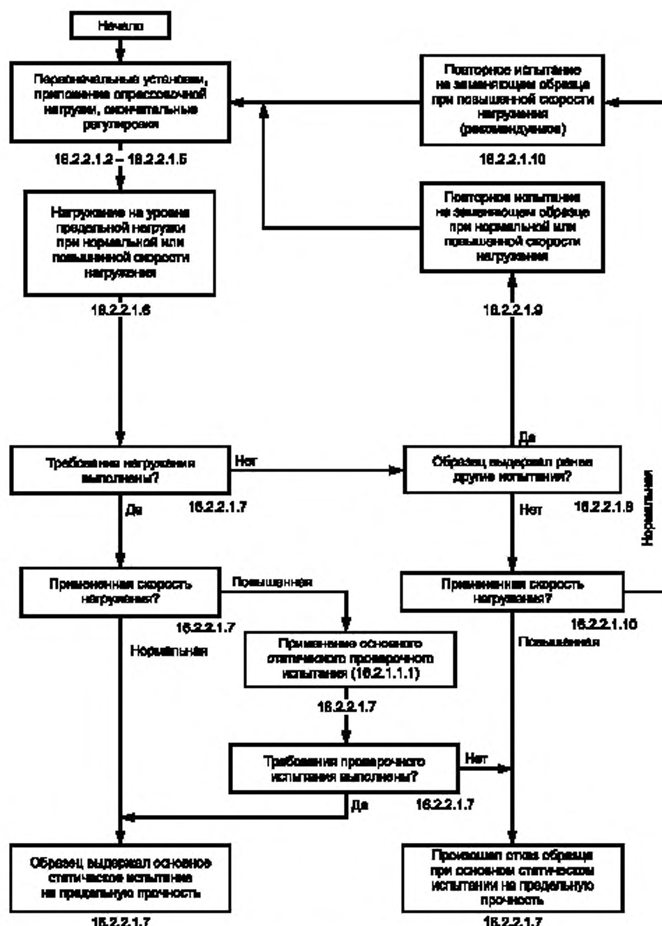
Рисунок 14 — Блок-схема основного статического испытания на предельную прочность, установленного в 18.2.2.1
