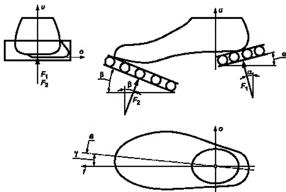
a — центральная линия узла стопы, соответствующая 6.7.2
