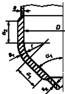
Рисунок 26 — Соединение обечайек с торидальным переходом
