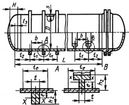
Рисунок 4 — Цилиндрическая обечайка, подкреплённая кольцами жесткости
