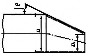
Рисунок 28 — Соединение кососимметричных обечайек
