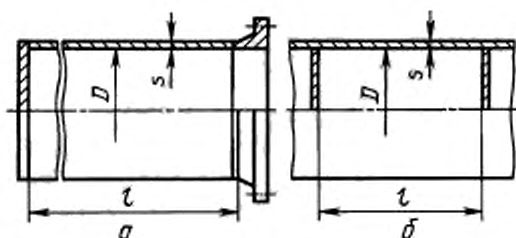
а — обечайка с фланцем или с плоским дном; б — обечайка с жесткими перегородками
