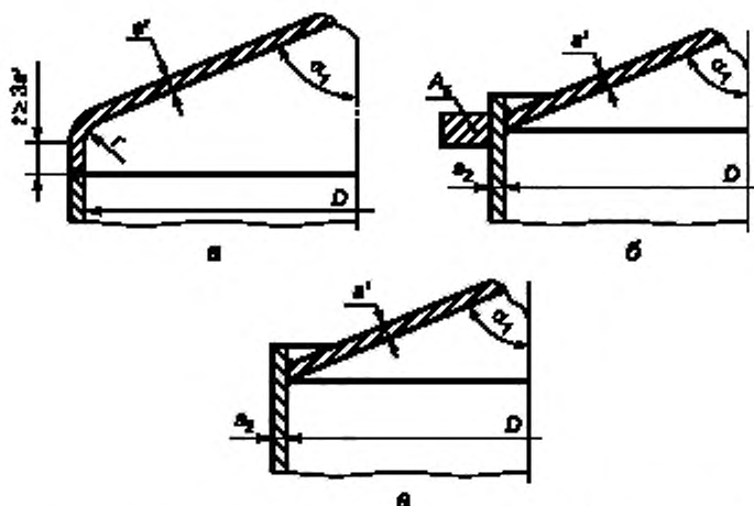
а — днище с торидальным переходом, б — днище с укрепляющим кольцом, в — днище без торидального перехода и укрепляющего кольца
