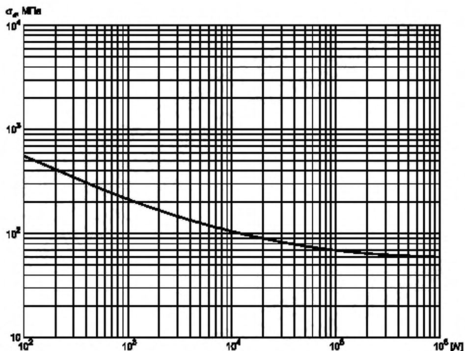
Рисунок 9 — Расчетная кривая усталости для сплава титана АТЗ (при A = 0,31 \cdot 10^5 МПа, B = 133,6 МПа, T = 350 °C)
