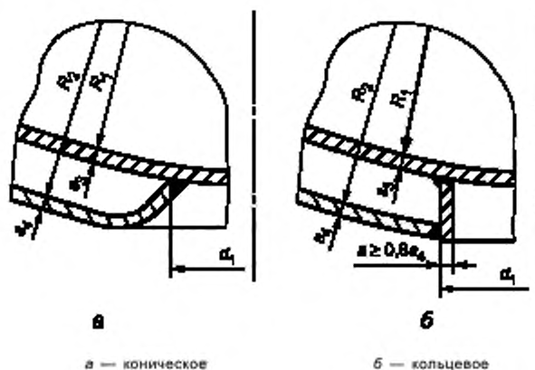
Рисунок А.3 — Сопряжение рубашки с дном
