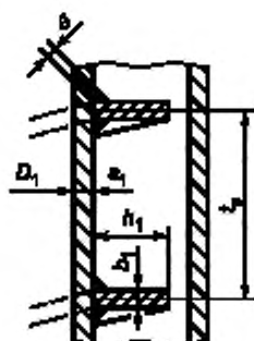
Рисунок А.6 — Направляющая спираль
