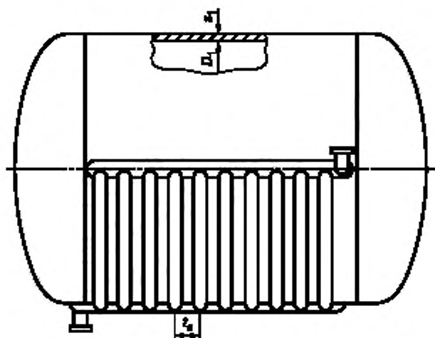
Рисунок А.9б — Сосуды с регистровыми каналами
