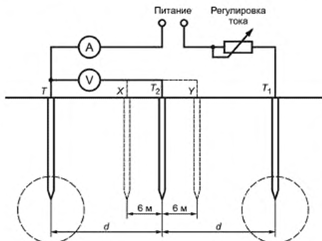
Зоны растекания (не перекрывающиеся)
