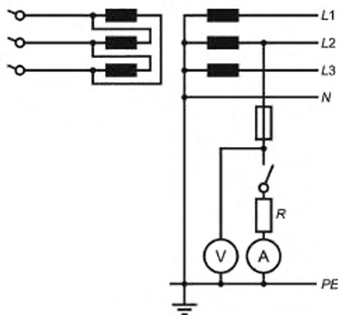
Рисунок D.1 — Схема измерения (метод 1)
