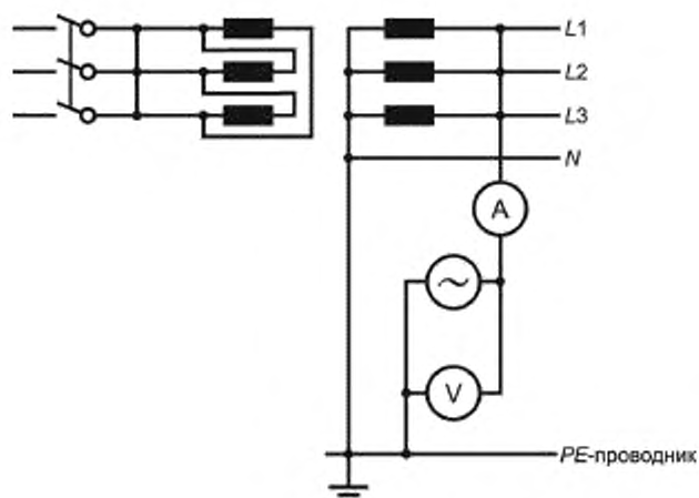
Рисунок D.2 — Схема измерения (метод 2)
