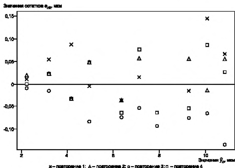
Рисунок 8 — Остатки и соответствующие значения \bar{y} в предположении о постоянстве стандартного отклонения остатков
