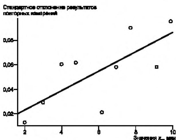
Рисунок 9 — Стандартные отклонения результатов повторных измерений для зазора между токопроводящими дорожками и значения x_0
