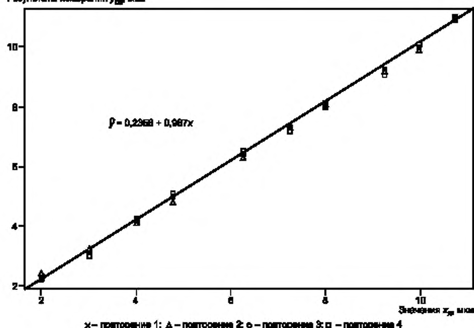
Рисунок 7 — Функция калибровки в предположении о постоянстве стандартного отклонения остатков
