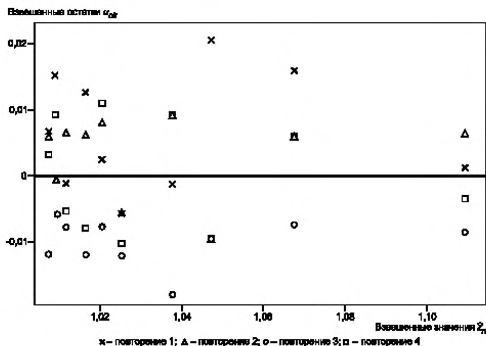
Рисунок 11 — Взвешенные остатки в зависимости от Z_n в предположении о пропорциональности стандартного отклонения остатков
