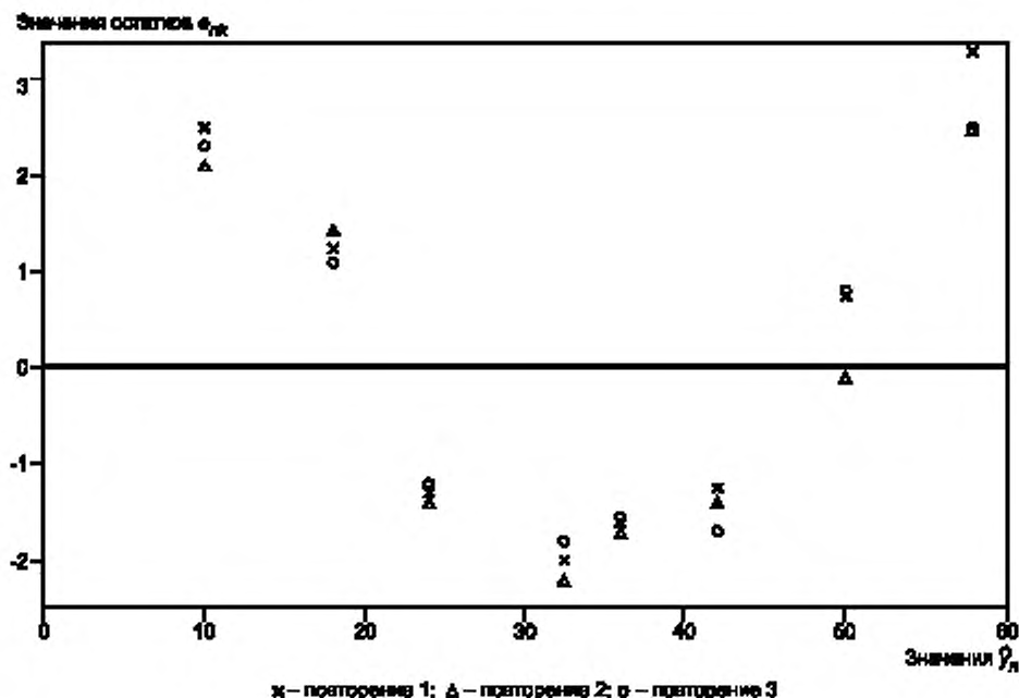
Рисунок 3 — График остатков как функция \hat{y}_n
