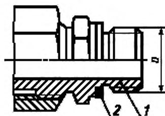
1 — ввертный конец корпусной детали, исполнение 1 по ГОСТ 22526; 2 — уплотнительная прокладка по ГОСТ 23358
