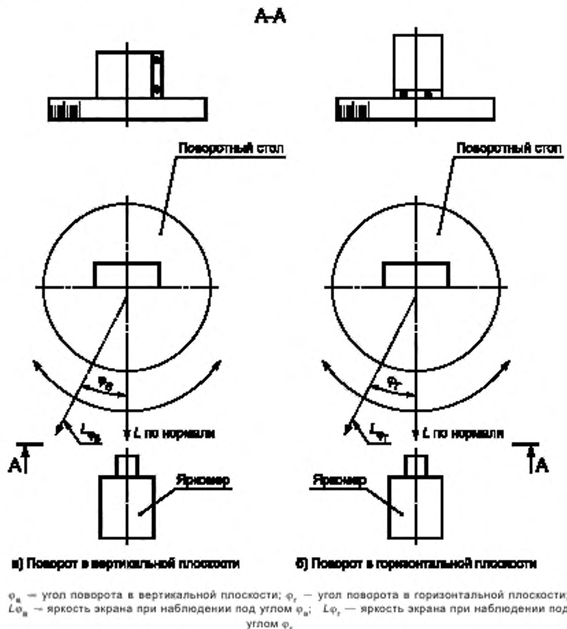
Рисунок 2 — Схема измерения зависимостей контраста и яркости изображения экрана или модуля СОИКП от угла наблюдения
