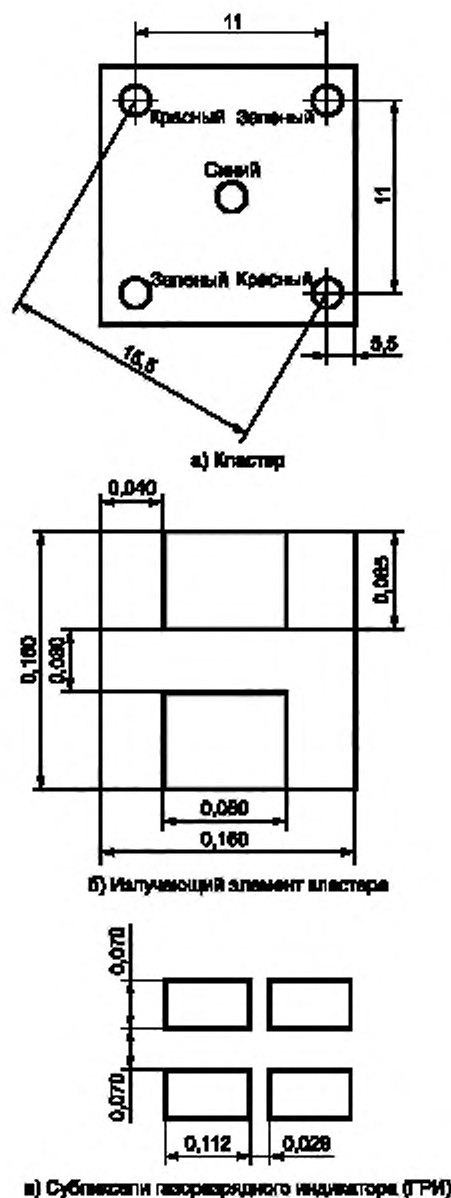
Рисунок 1 — Возможные варианты излучающих источников в экранах СОИКП
