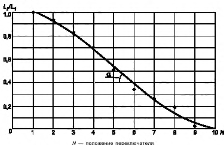
Рисунок 4 — Изменение яркости излучения экранов от регулировки
