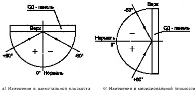
а) Измерение в азимутальной плоскости б) Измерение в меридиональной плоскости
