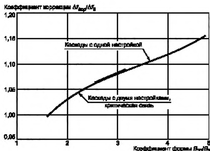
Рисунок Д.1 — Коэффициент коррекции для оценки отношения B_{дв}/B_{ср} для других типов настраиваемых схем
