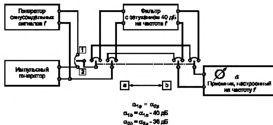
Рисунок 3 — Схема измерения ослабления продуктов интермодуляции
