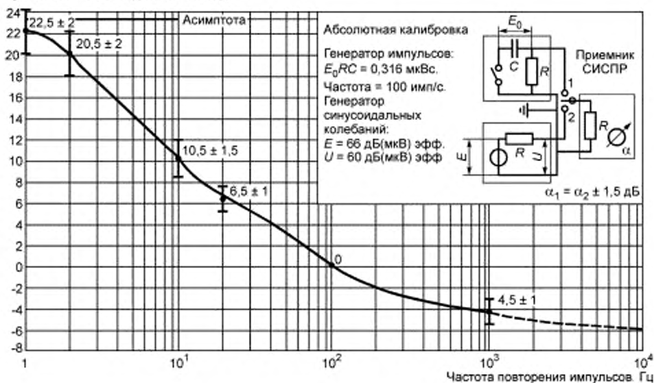
б) Импульсная характеристика ИП для полосы частот В (от 0,15 до 30 МГц) и допускаемые отклонения ее значений
