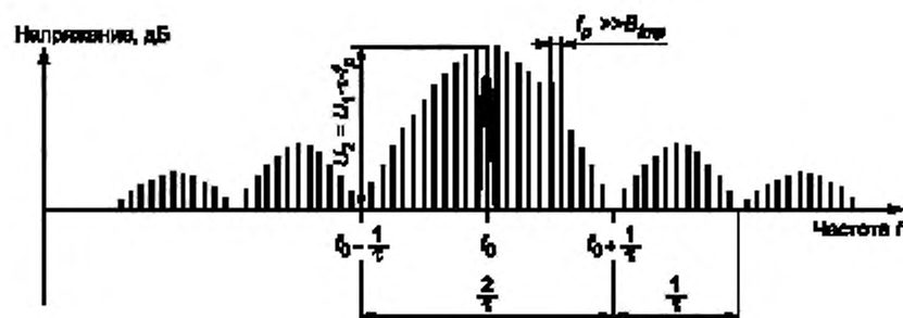
Рисунок Д.5 — Фильтрация в случае, если значение B_{\text{имр}} намного меньше частоты повторения импульсов
