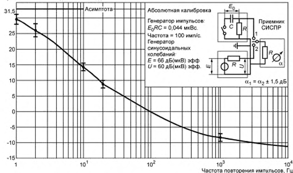
в) Импульсная характеристика ИП для полосы частот С/Д (от 30 до 1000 МГц) и допускаемые отклонения ее значений
