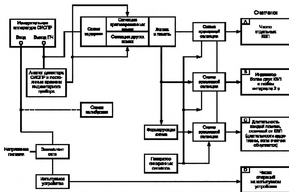
Рисунок 6 — Пример блок-схемы анализатора кратковременных ИРП
