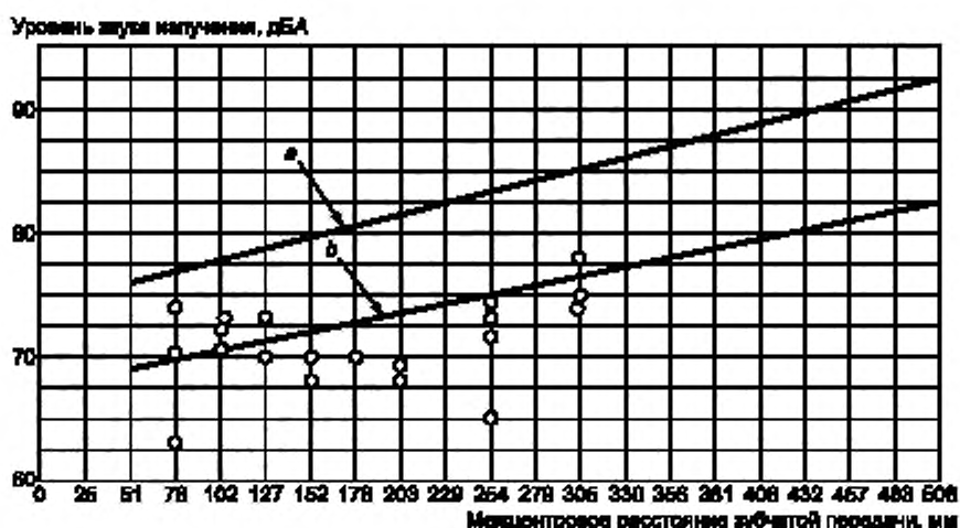
Рисунок В.7 — Уровень звука излучения одноступенчатого червячного редуктора с охлаждающим вентилятором при частоте вращения входного вала 1750 об/мин на расстоянии 1,5 м от корпуса на холостом ходу или при малой нагрузке в зависимости от межцентрового расстояния
