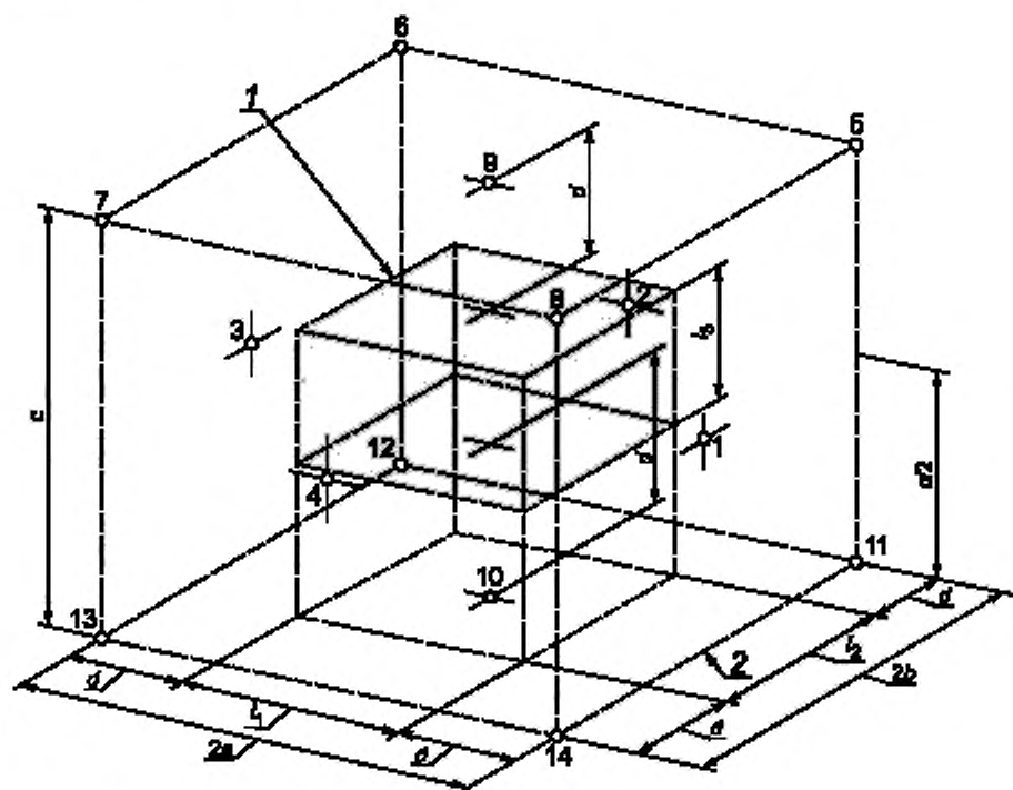
1 — гибящий параллелепипед; 2 — измерительная поверхность
