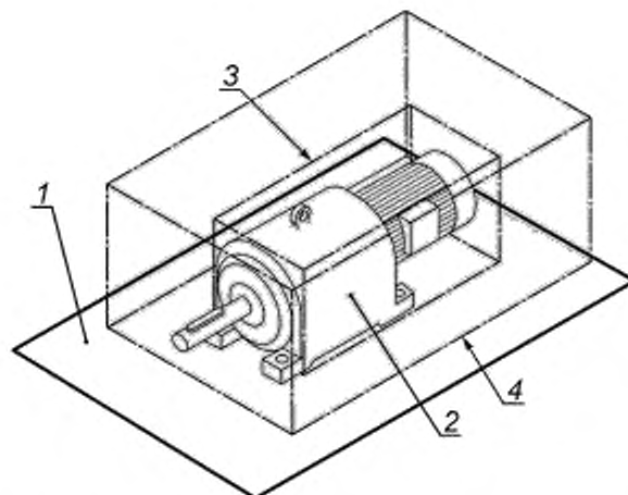
1 — пол; 2 — редуктор; 3 — огибающий параллелепипед; 4 — измерительная поверхность
