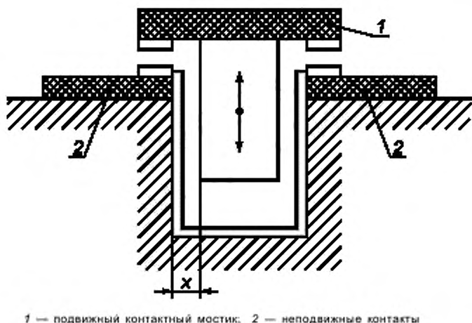
Рисунок G.2 — Расстояние утечки между подвижными и неподвижными контактодержателями из изоляционного материала
