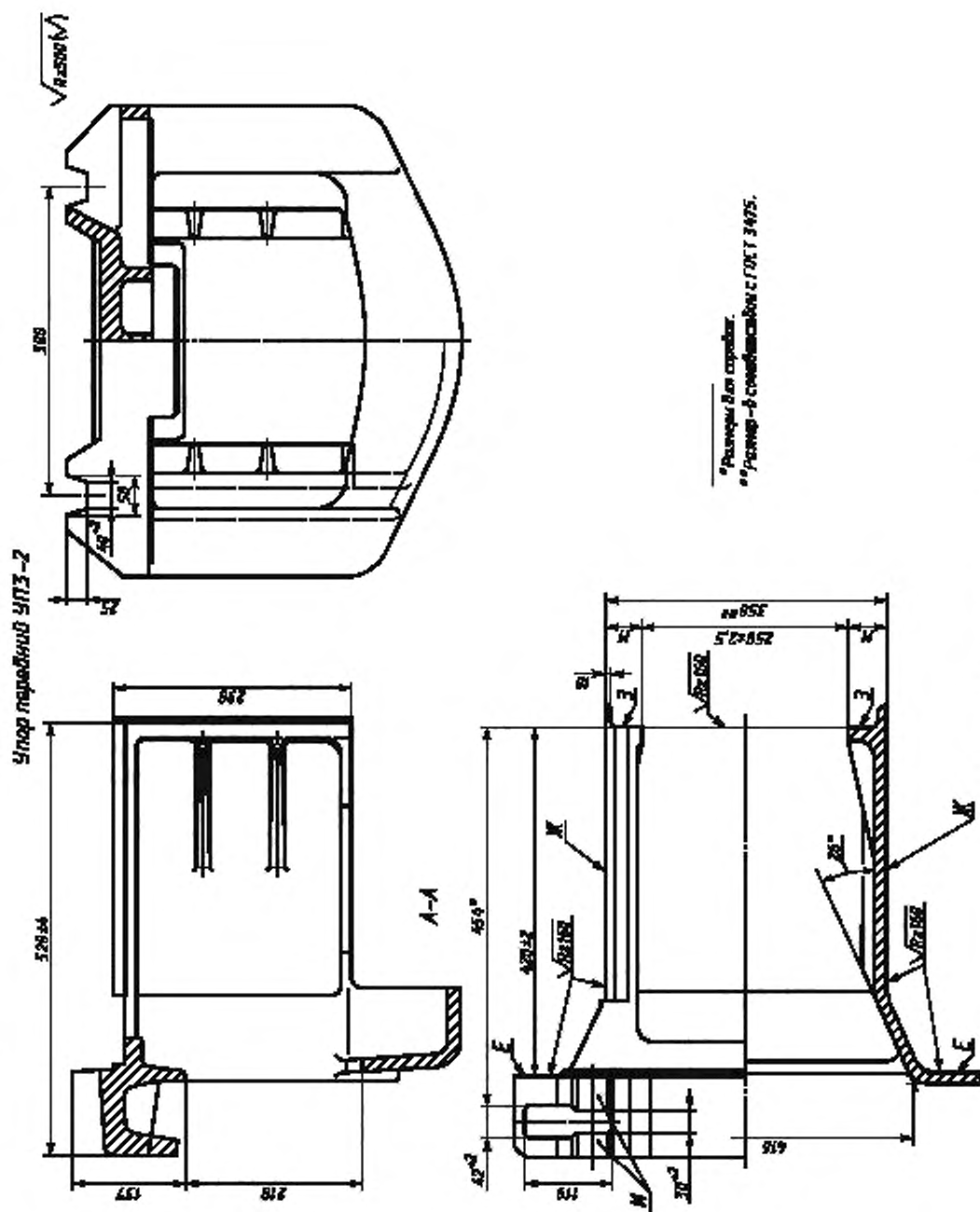
Рисунок 5 — Упор передний УПЗ-2
