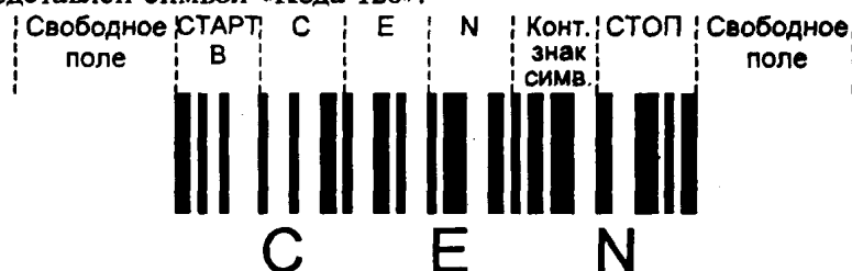
Рисунок 1 — Символ «Кода 128», кодирующий знаки CEN
