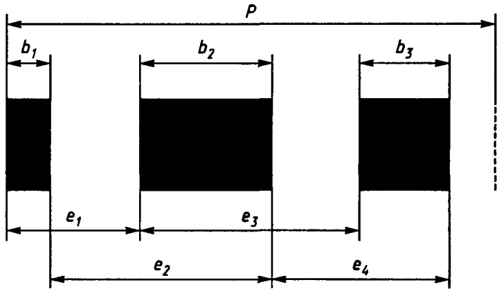
Рисунок 4 — Размеры для допусков
