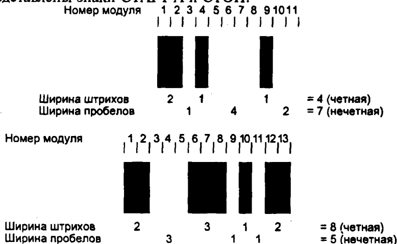
Рисунок 2 — Знаки СТАРТ А и СТОП в «Код 128»
