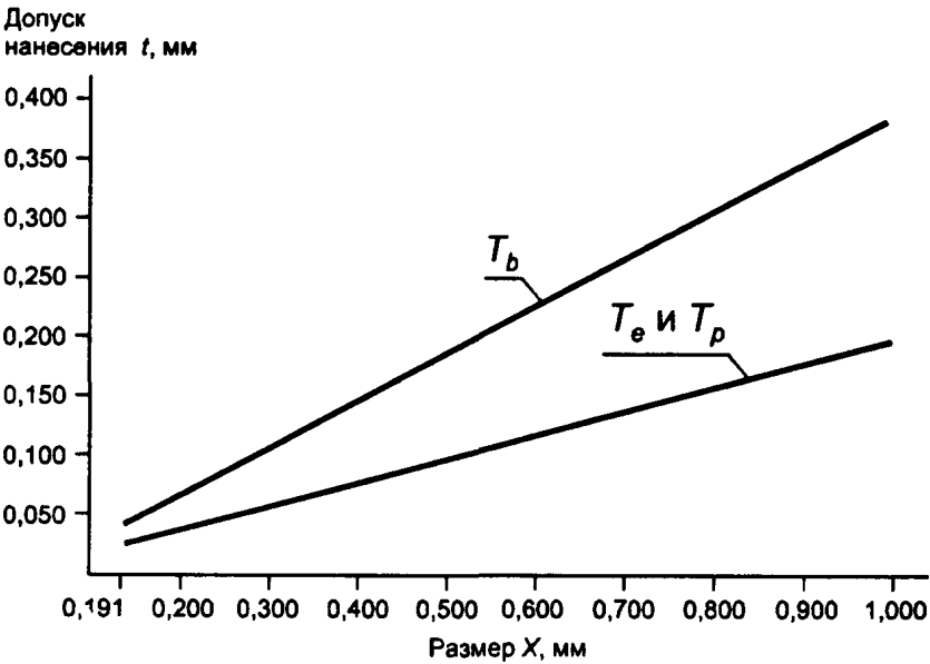
Рисунок 5 — Допуски для «Кода 128»
