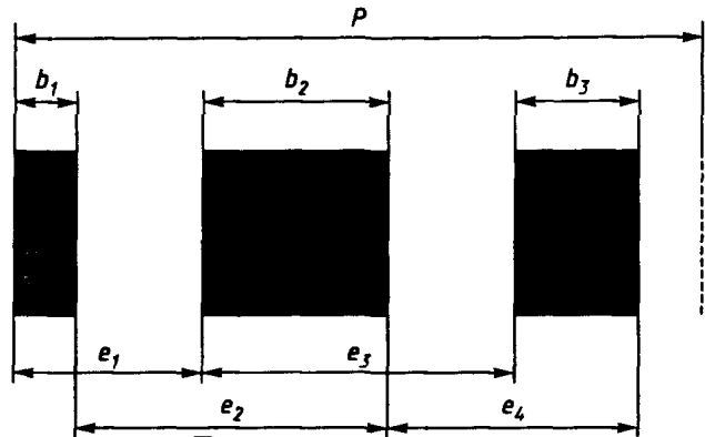
Рисунок 6 — Размеры для декодирования
