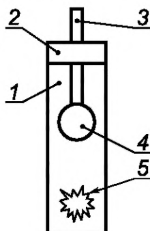
1 — реакционная пробирка; 2 — пробка; 3 — стеклянная палочка; 4 — реагент на стеклянном шарике; 5 — измельченный образец кожной ткани или волоса
