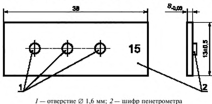
Рисунок Б.1 — Стандартный пластинчатый пенетromетр
