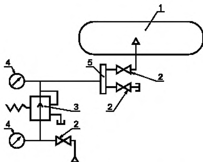
Рисунок Б.2 — Стенд пневматических испытаний
