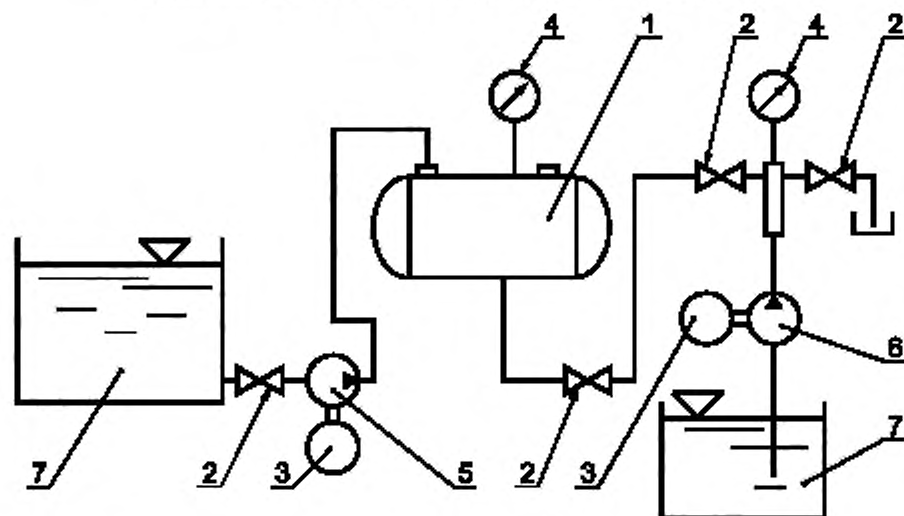
Рисунок Б.1 — Стенд гидравлических испытаний
