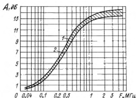
1 — верхний предел характеристики предельных при T = 1,35 мкс и X = 4,3 ; 2 — нижний предел характеристики предельных при T = 1,25 мкс и X = 3,7
