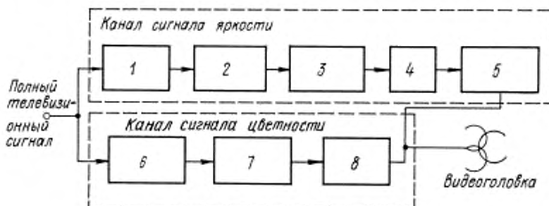
1, 8 — фильтры нижних частот; 2 — схема частотных предсказаний; 3 — частотный модулятор; 4 — фильтр верхних частот; 5 — усилитель записи; 6 — полосовой фильтр; 7 — делитель частоты на четыре
