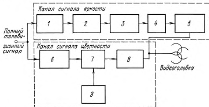
1, 8 — фильтры нижних частот; 2 — схема частотных предсказаний; 3 — частотный модулятор; 4 — фильтр верхних частот; 5 — усилитель записи; 6 — полосовой фильтр; 7 — преобразователь частоты; 9 — гетеродин
