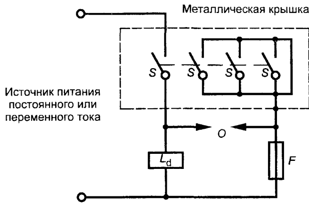
Обозначения к рисункам 5 и 6 L d — нагрузка по схеме рисунка 7, F — предохранитель, O — датчик перенапряжения (см. 8.3.3.5.4), S — коммутирующий элемент (нормально разомкнутый или нормально замкнутый)
