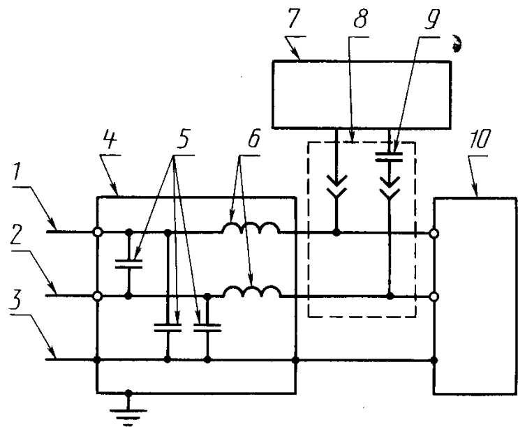
1, 2, 3 — фазный, нейтральный и защитный провода сети электропитания соответственно; 4 — устройство развязки; 5 — конденсаторы развязки; 6 — индуктивности развязки; 7 — ИГ МИП; 8 — устройство связи; 9 — конденсатор связи; 10 — ИТС
