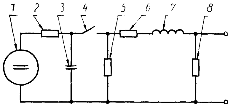
Упрощенная схема ИГ МИП
