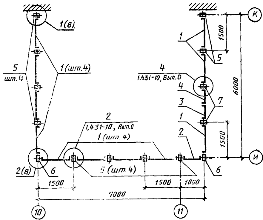
Пример выполнения схемы расположения элементов сборных перегородок Схема ...
