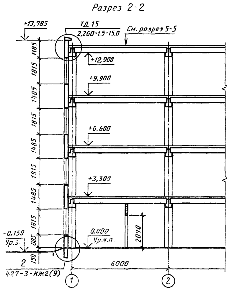
Пример выполнения разреза многоэтажного производственного здания
