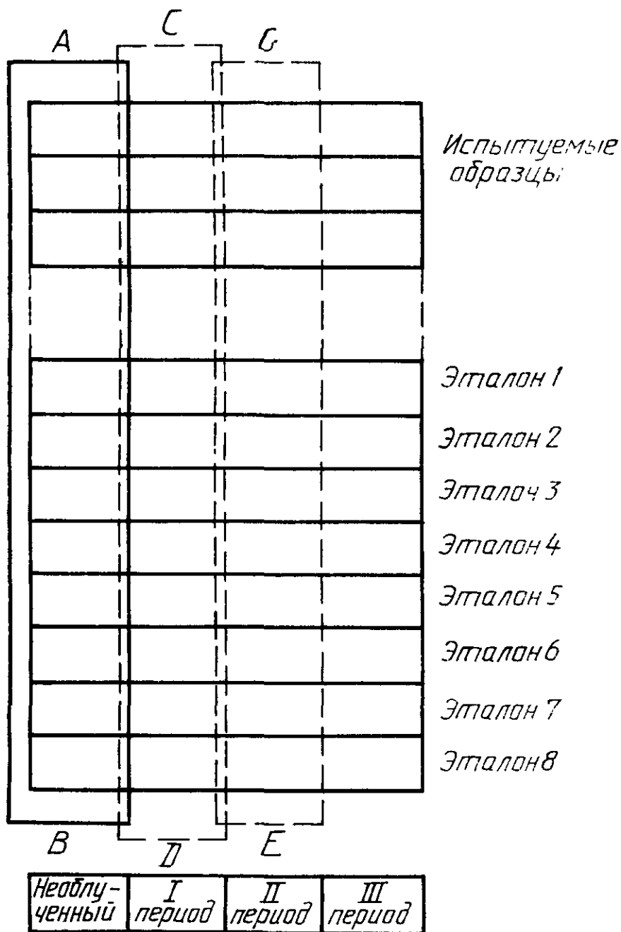
Схема расположения испытуемых образцов и синих эталонов
