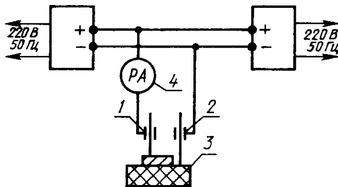
1, 2 — цанговый зажим; 3 — платиновые сетчатые электроды (комплект); 4 — амперметр
