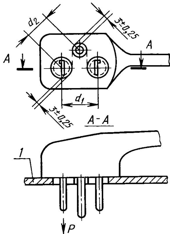
1 — стальная пластина Черт. 34
