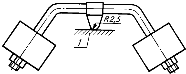
1 — образец Черт. 35
