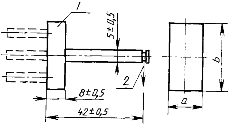
1 — материал (сталь); 2 — прилагаемая сила
