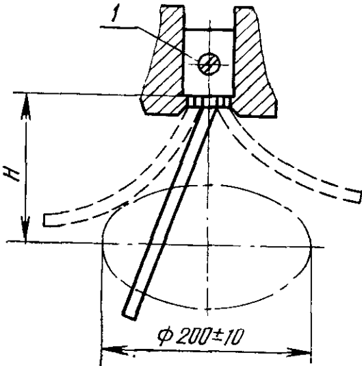
1 — зажим
